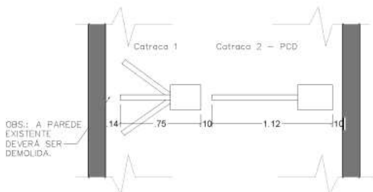
PLANTA BAIXA - PÁTIO FINANÇAS (RAMPA)
