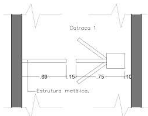
PLANTA BAIXA - FINANÇAS (ESCADA)
